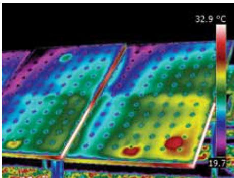
Diese roten Stellen zeigen Module an, die ständig wärmer sind als der Rest, und liefern somit einen Hinweis auf fehlerhafte Anschlüsse.
