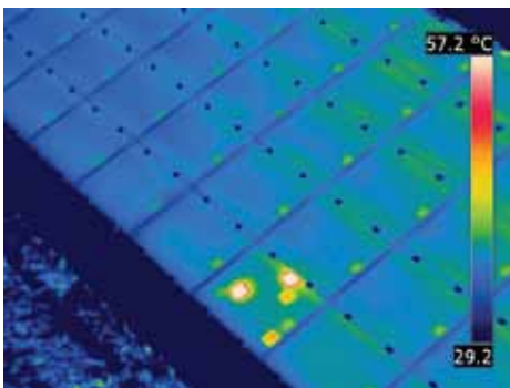
Dieses Wärmebild zeigt ein Beispiel für ein sogenanntes "Patchwork-Muster", das bei einer fehlerhaften Bypass-Diode der Solarzelle erscheint.
